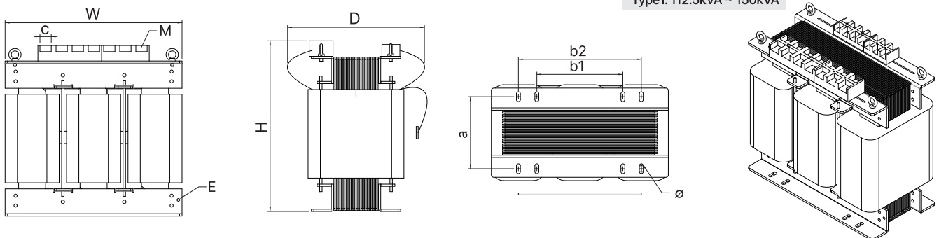
Type2. 175kVA ~ 325kVA
